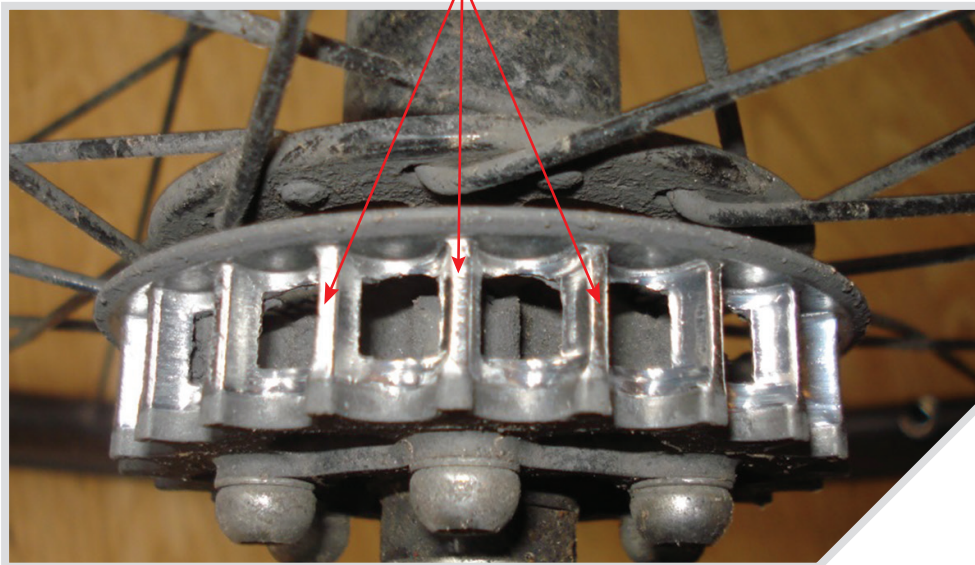
Versleten CDC-tandwieltanden
