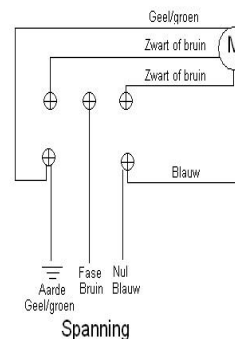
Aansluitschema Presto en Geba Schakelaar
